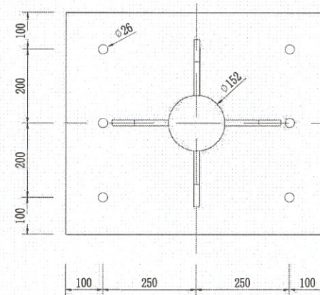
底座法兰盘
