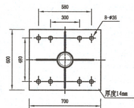
B-B剖视图
